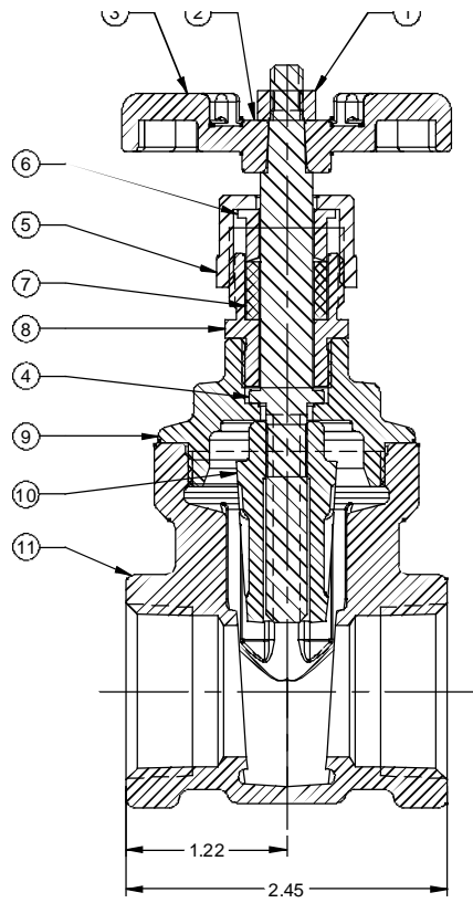
SECTION A-A
